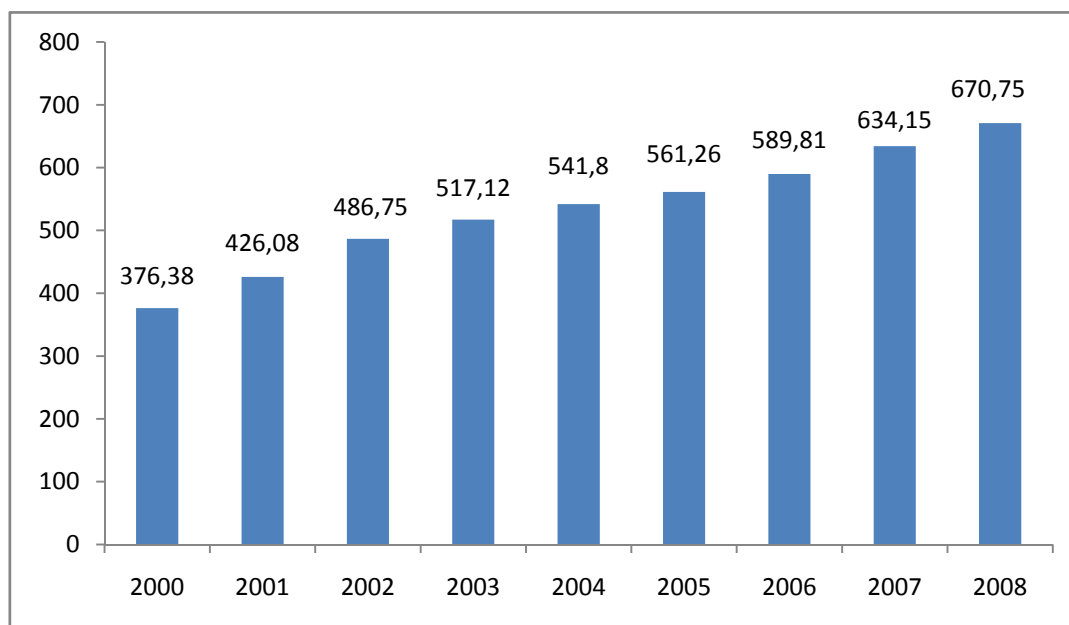
Graphique 2.3 : Consommation d'énergie électrique de 2000 à 2008 au Bénin (en MWh)
